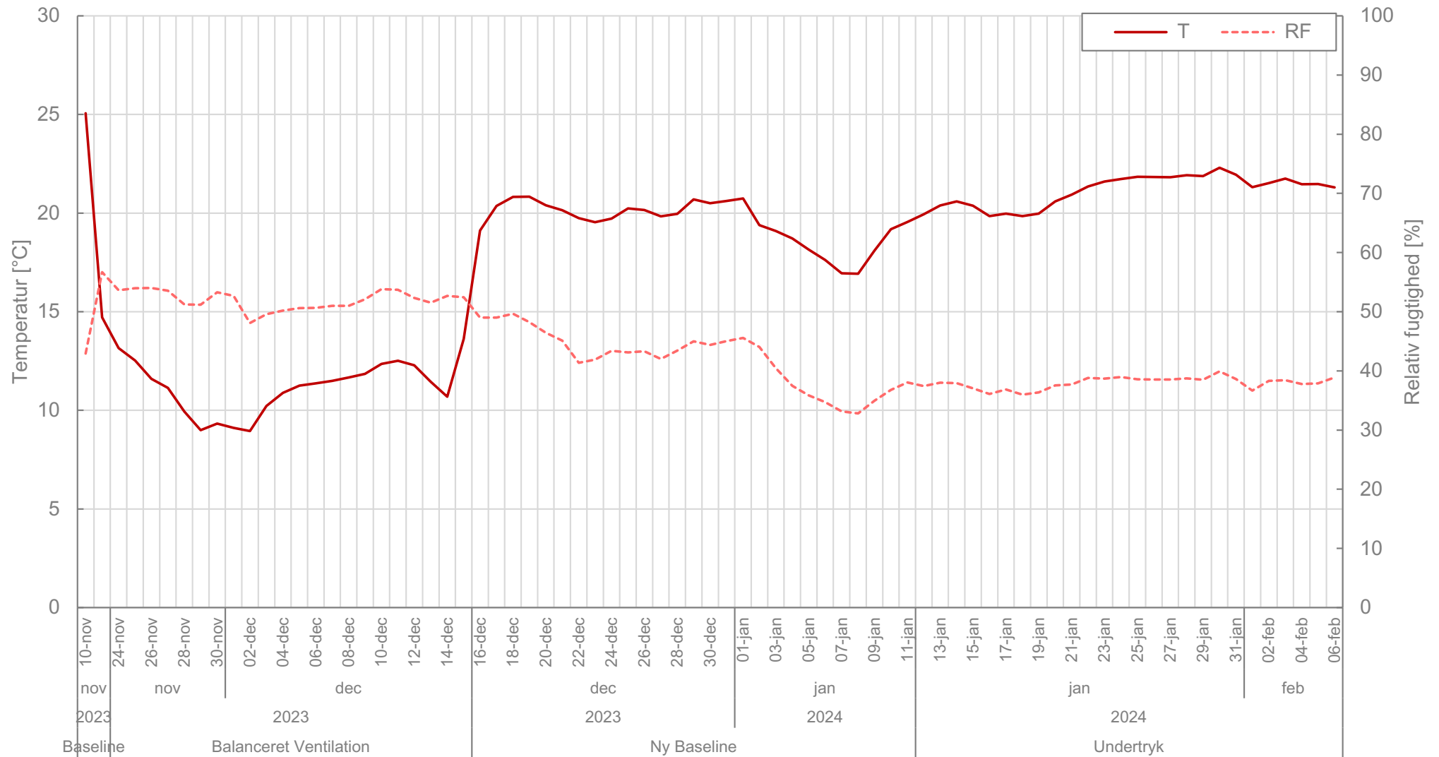
Bilag 17: Smartlogger (SL2) Træfugt på gulv ved T8 og T10 10/11 2023 til 5/2 2024
