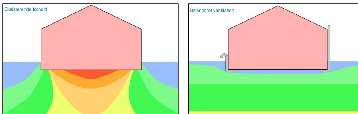
Figur 5: Vintersituation hhv. uden og med balanceret ventilation
