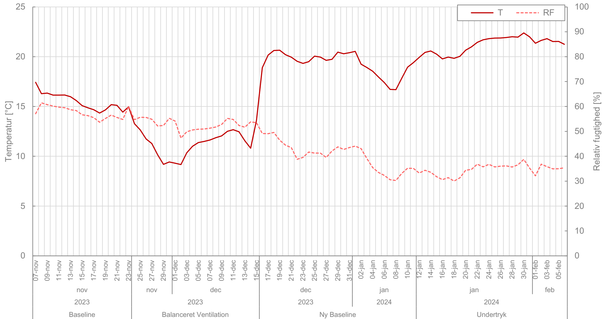
Bilag 12: T10 (V10-24) - Temperatur og fugt på gulv 7/11 2023 til 5/2 2024
