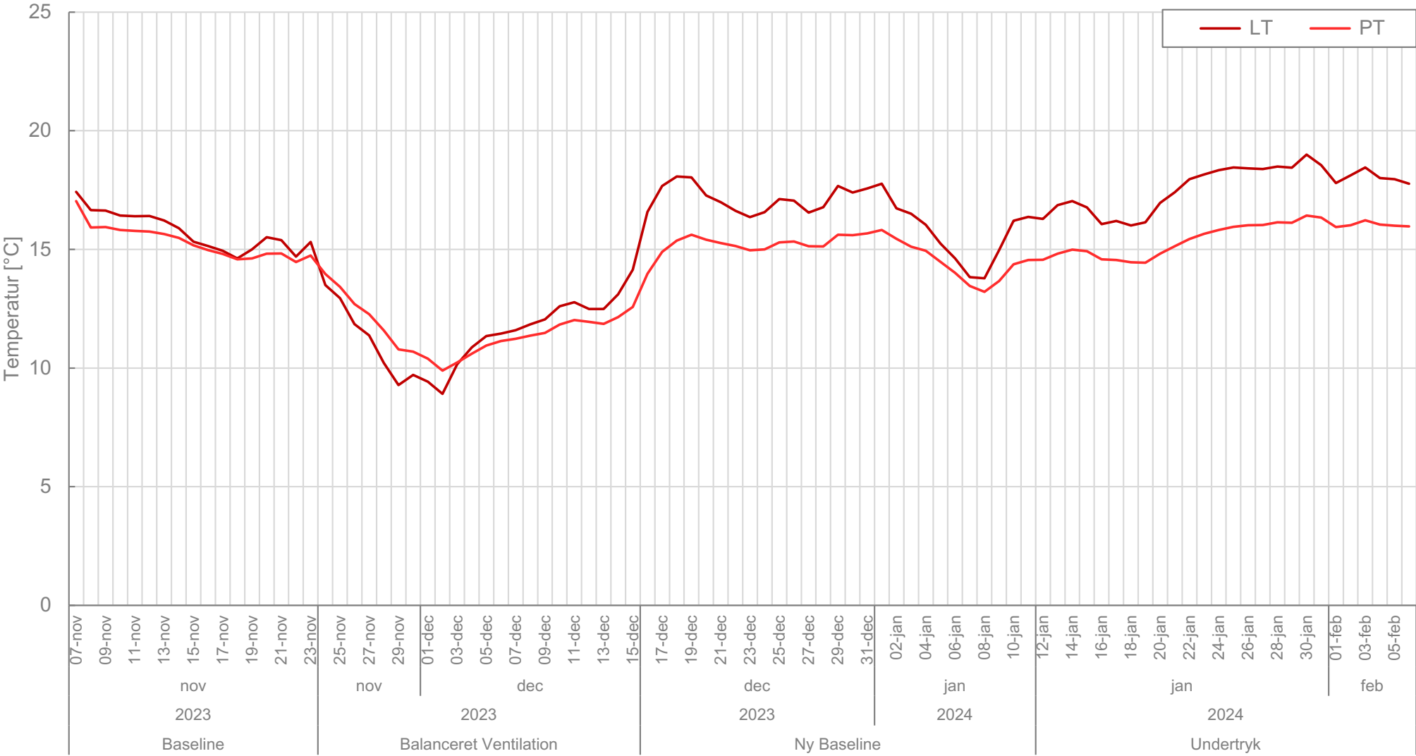
Bilag 7: T5 (ARH-1-06) - Temperatur på og under gulv 7/11 2023 til 5/2 2024
