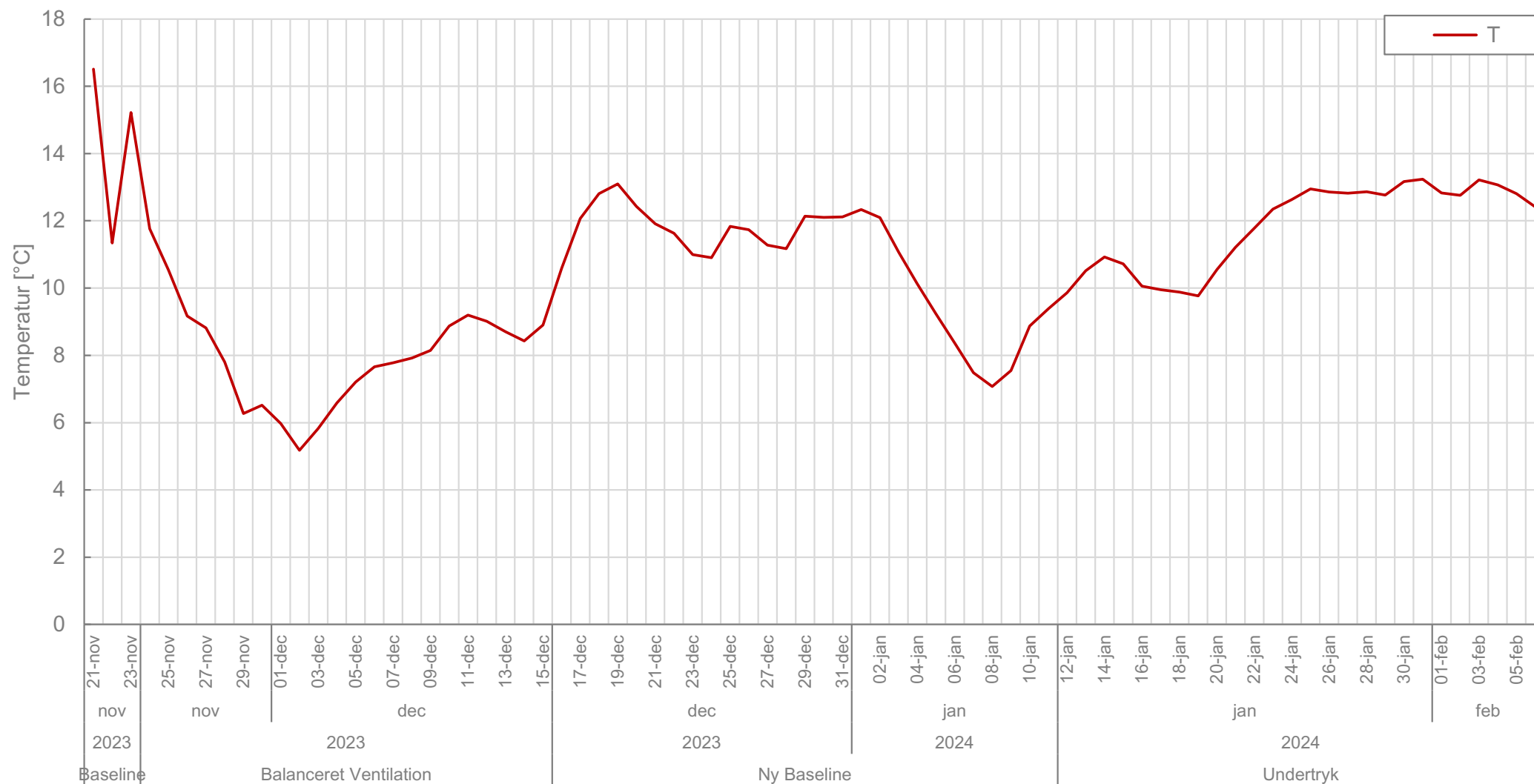
Bilag 5: T3 (V12-03) - Temperatur under gulv 23/11 2023 til 5/2 2024
