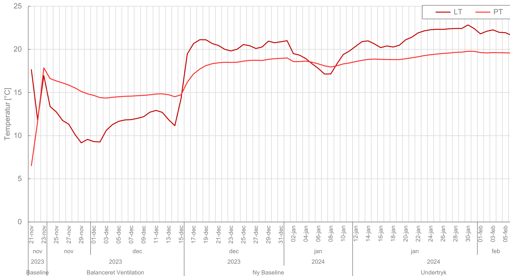
Bilag 10: T8 (V10-27) - Temperatur på og under gulv 23/11 2023 til 5/2 2024
