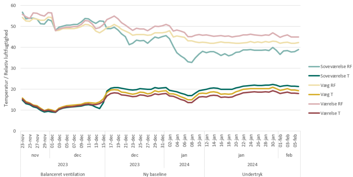
Figur 17: temperatur og fugt på træoverflader. Trægulv værelse ved T6 (SL1), trægulv soveværelse ved T8 (SL2) og trævæg mellem T6 og T8 (SL3).
