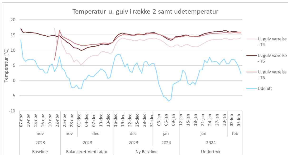
Figur 15: Række 2 (jordtemperatur, T4, T5 og T6) i forhold til udeluft (T11)
