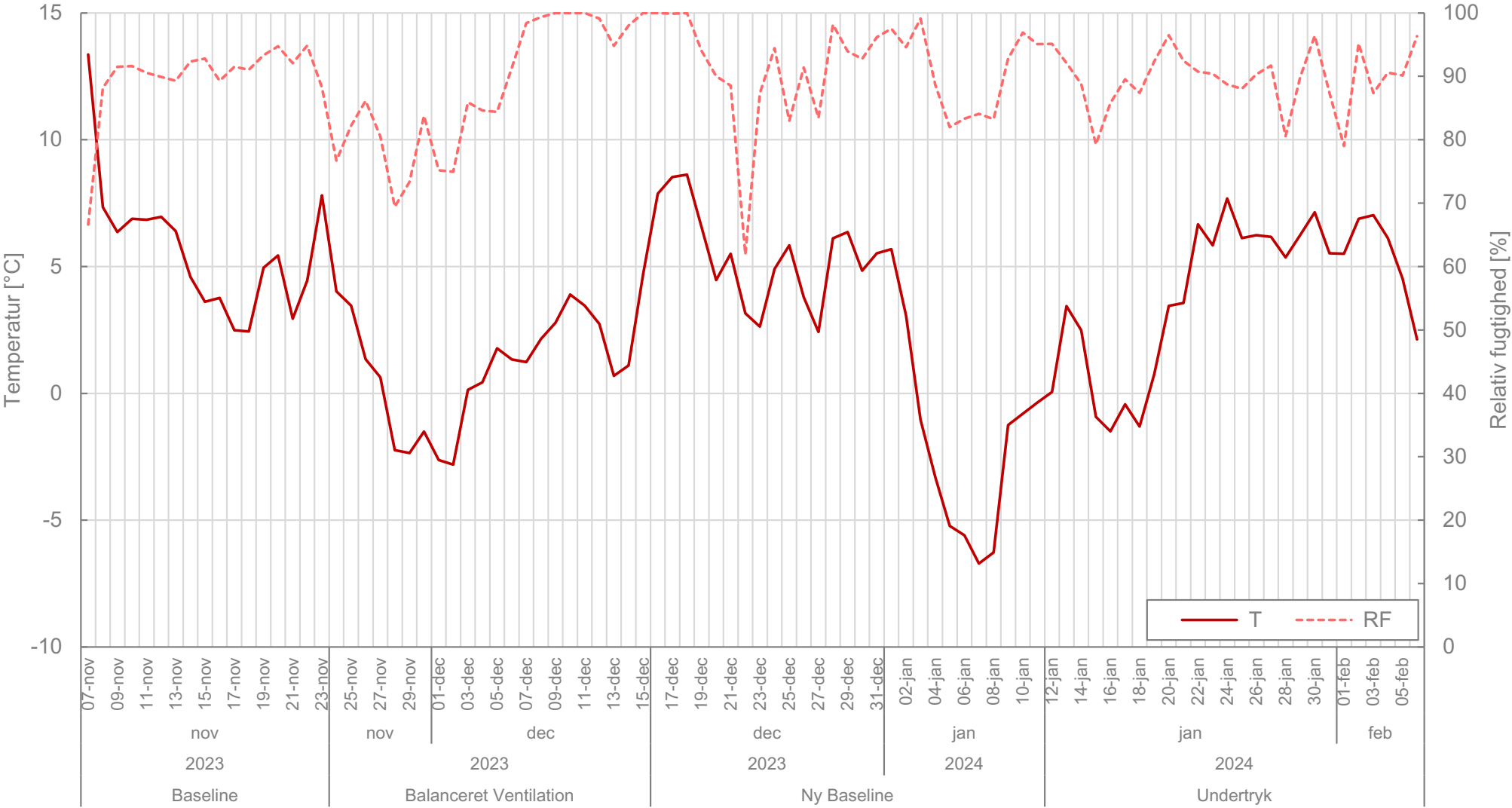
Bilag 13: T11 (V10-22) - Temperatur og fugt udeluft 7/11 2023 til 5/2 2024
