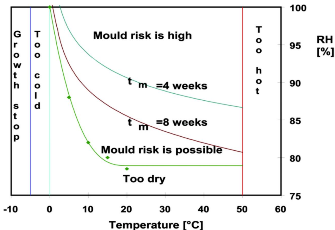
Figur 20: Vækstbetingelser for skimmelsvamp i træmaterialer (Ref. /1/).
