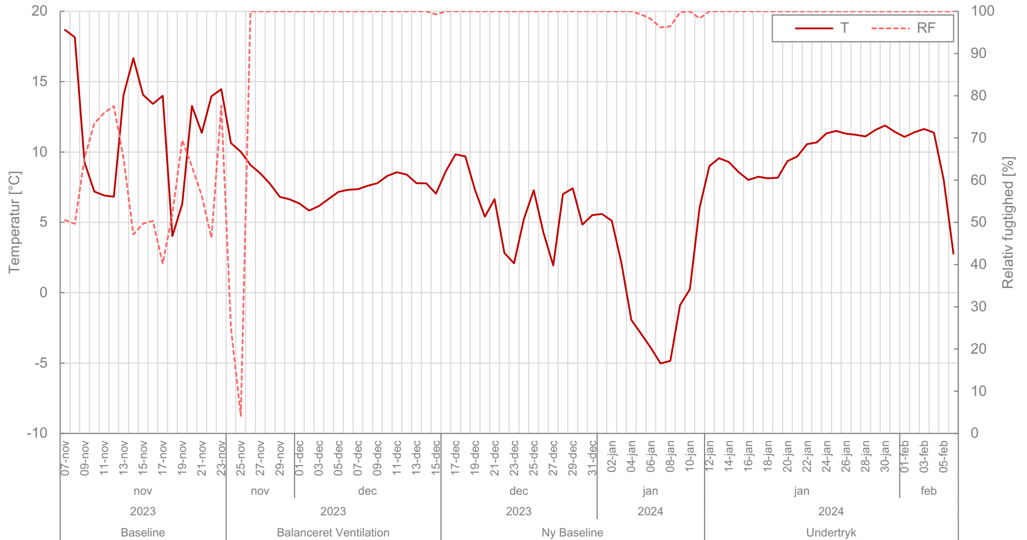
Bilag 14: T12 (V10-23) - Temperatur og fugt afkastluft 7/11 2023 til 5/2 2024
