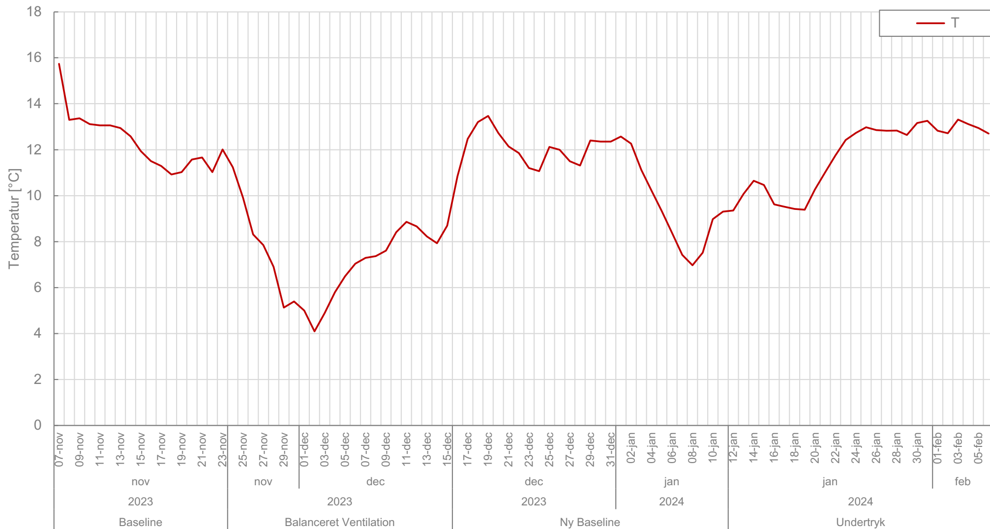
Bilag 4: T2 (V12-01) - Temperatur under gulv 7/11 2023 til 5/2 2024
