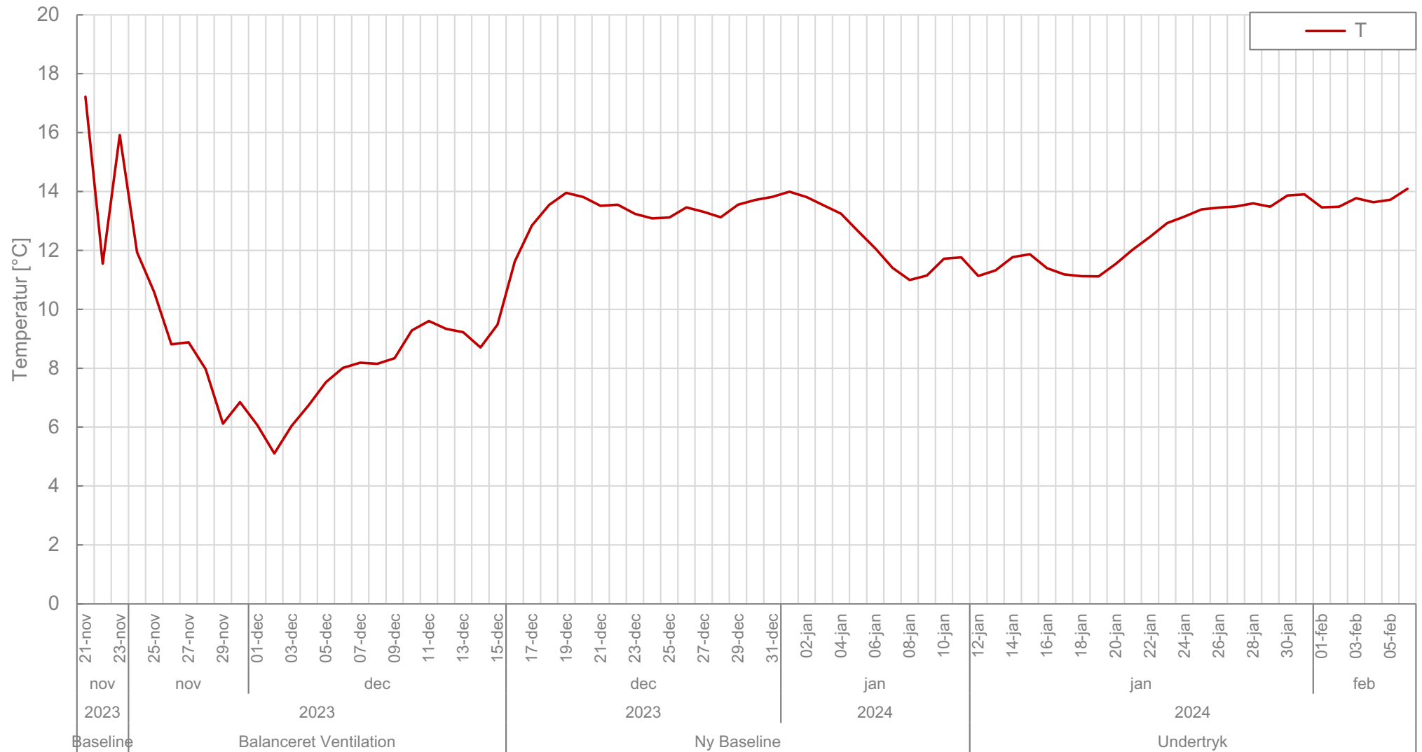
Bilag 6: T4 (12-02) - Temperatur under gulv 23/11 2023 til 5/2 2024
