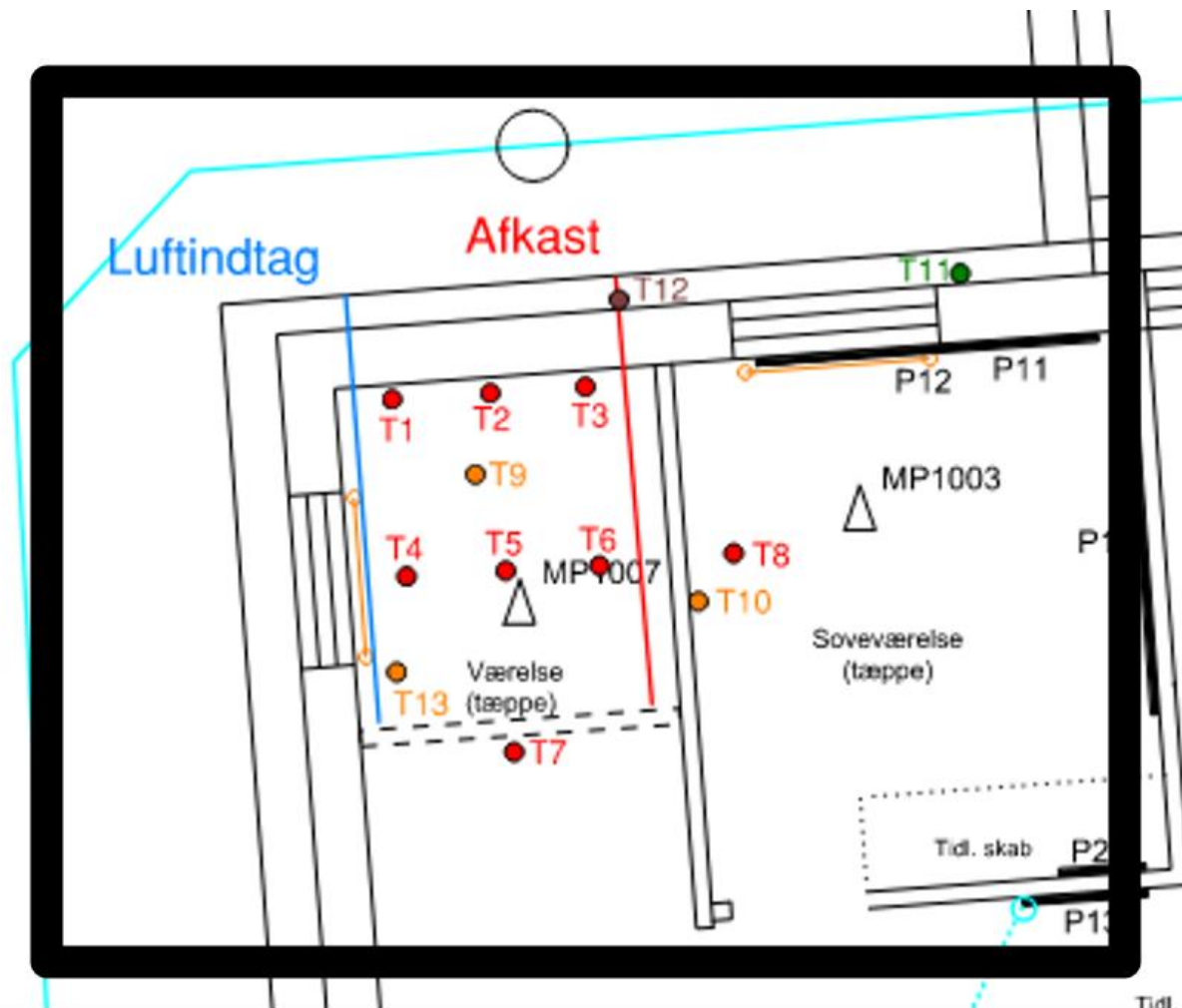
Figur 11: Forstørrelse af "projektområdet". Placering af målepunkter og ventilationsstrengene.
