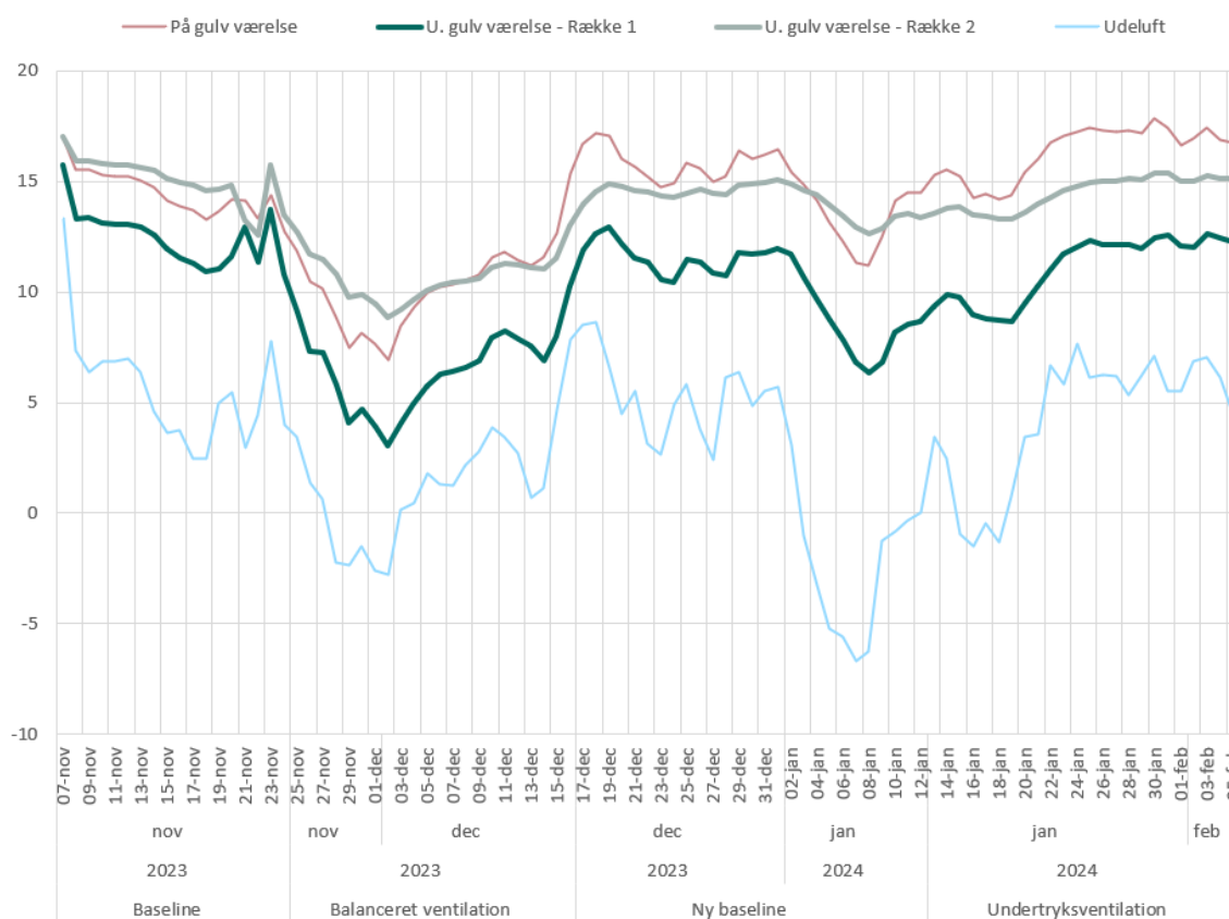
Figur 14: Temperatur under gulv i række 1 og 2 og på gulv, sammenholdt med udeluft-temperatur.
