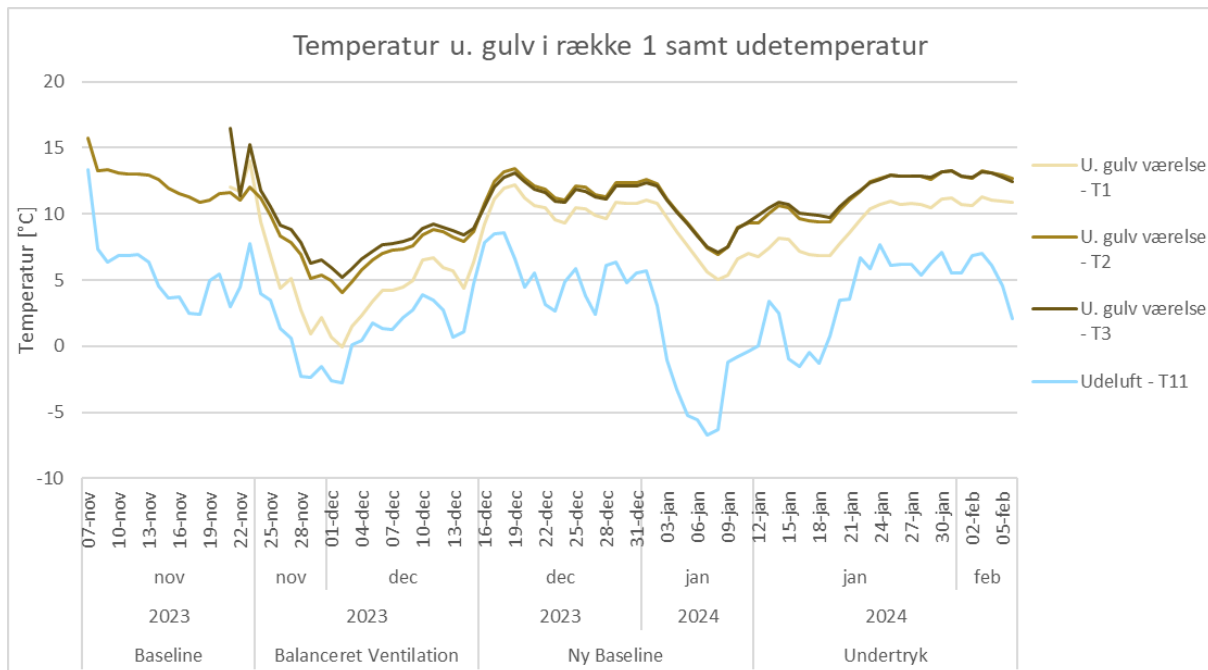
Figur 16: Række 1 (jordtemperatur, T1, T2 og T3) i forhold til udeluft (T11)
