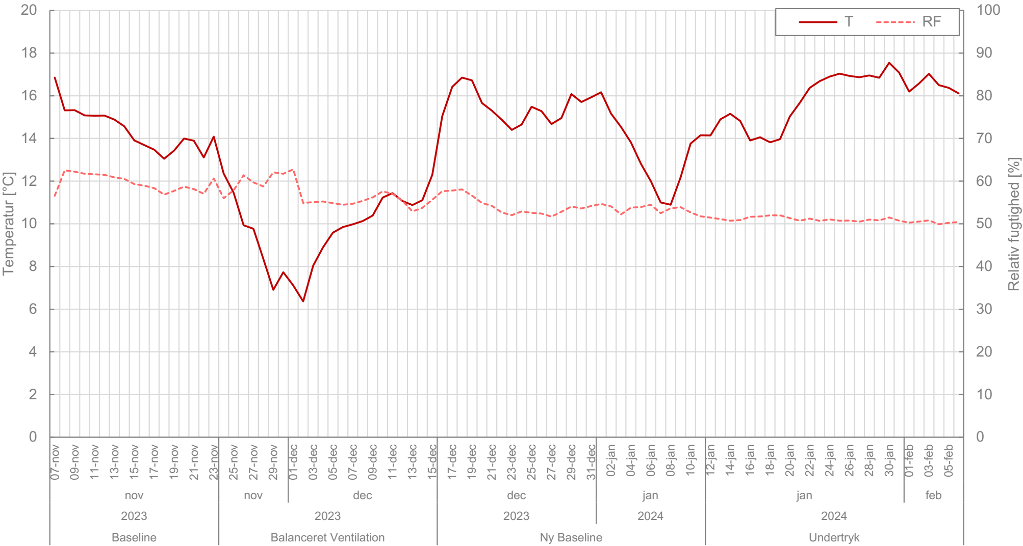
Bilag 15: T13 (ARH-1-04) - Temperatur og fugt på gulv 7/11 2023 til 5/2 2024
