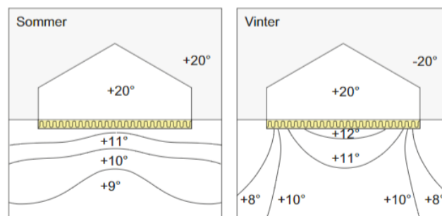
Figur 4: Temperaturforhold i jord jf. SBI-anvisning 279, ref. /2/. Reproduceret med tilladelse fra BUILD, Aalborg Universitet.
