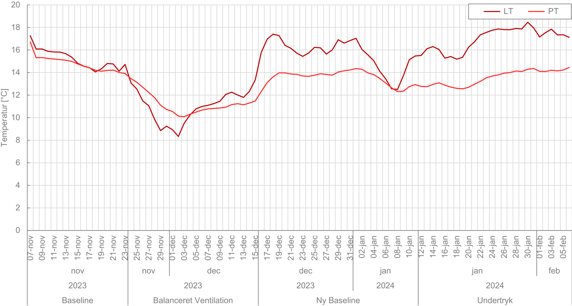
Bilag 9: T7 (ARH-1-05) - Temperatur på og under gulv 7/11 2023 til 5/2 2024
