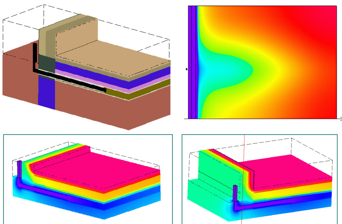
Figur 3: Eksempler på simulering med HEAT-3 ved tilførsel af kold luft under gulv – både opbygning af model og temperaturforskellene på gulv og op gennem gulvkonstruktionen.
