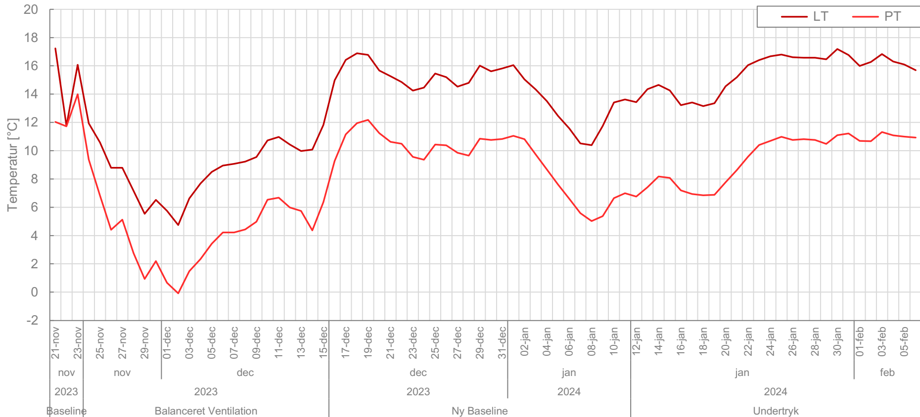
Bilag 3: T1 (V10-29) - Temperatur på og under gulv 23/11 2023 til 5/2 2024
