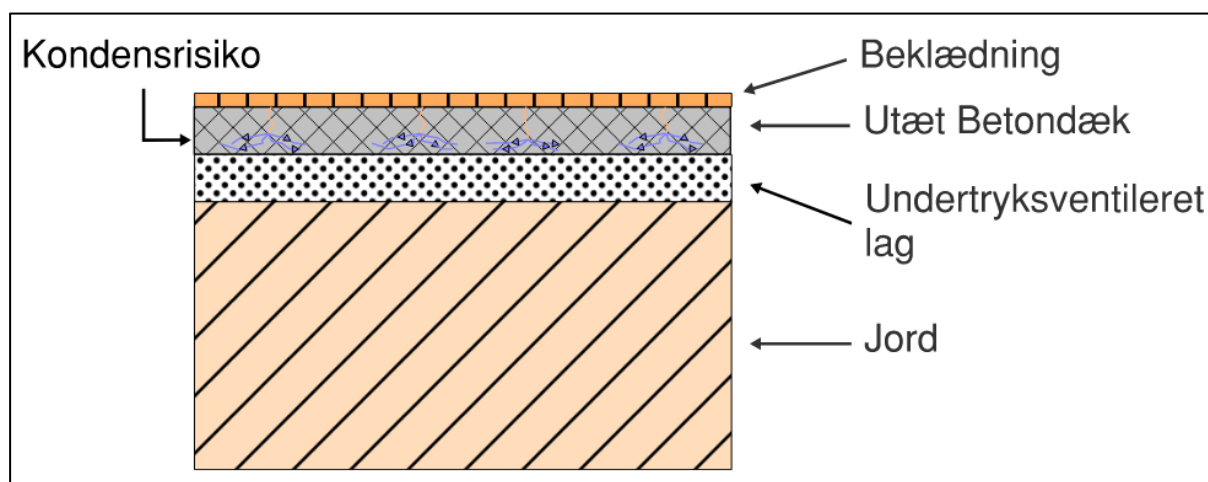
Figur 2: Kondensrisiko ved undertryksventilation i TESTHUSET. Ved denne figur ses den aktuelle gulvopbygning, hvor der ved undertryksventilation trækkes varm fugtig luft ned i betondækket.
