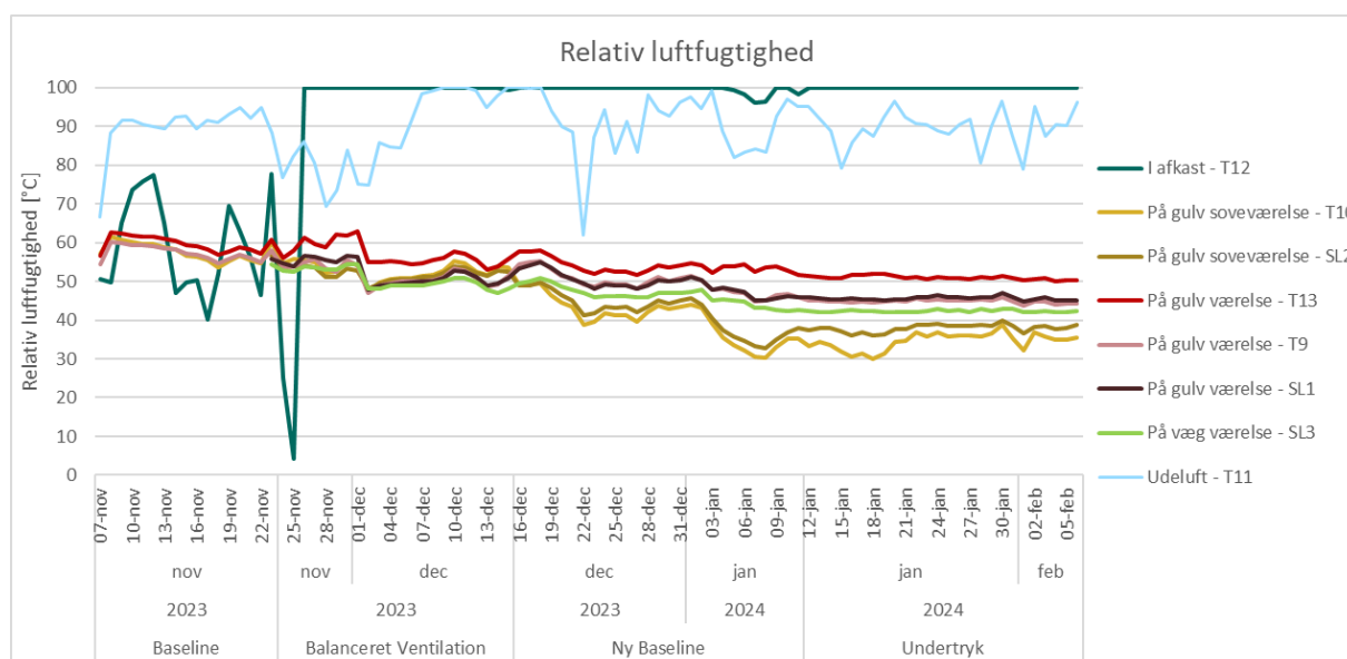
Figur 18: Relativ luftfugtighed for målere med RF-sensor.
