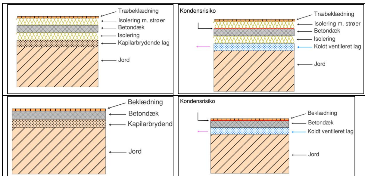
Figur 1: Problematiske gulvkonstruktioner ved balanceret ventilation under gulv. Øverst ses en situation, hvor der er isolering over og under et betondæk, mens situationen nederst viser den aktuelle situation i TESTHUSET, hvor der ikke er isolering, hverken over eller under betondækket.
