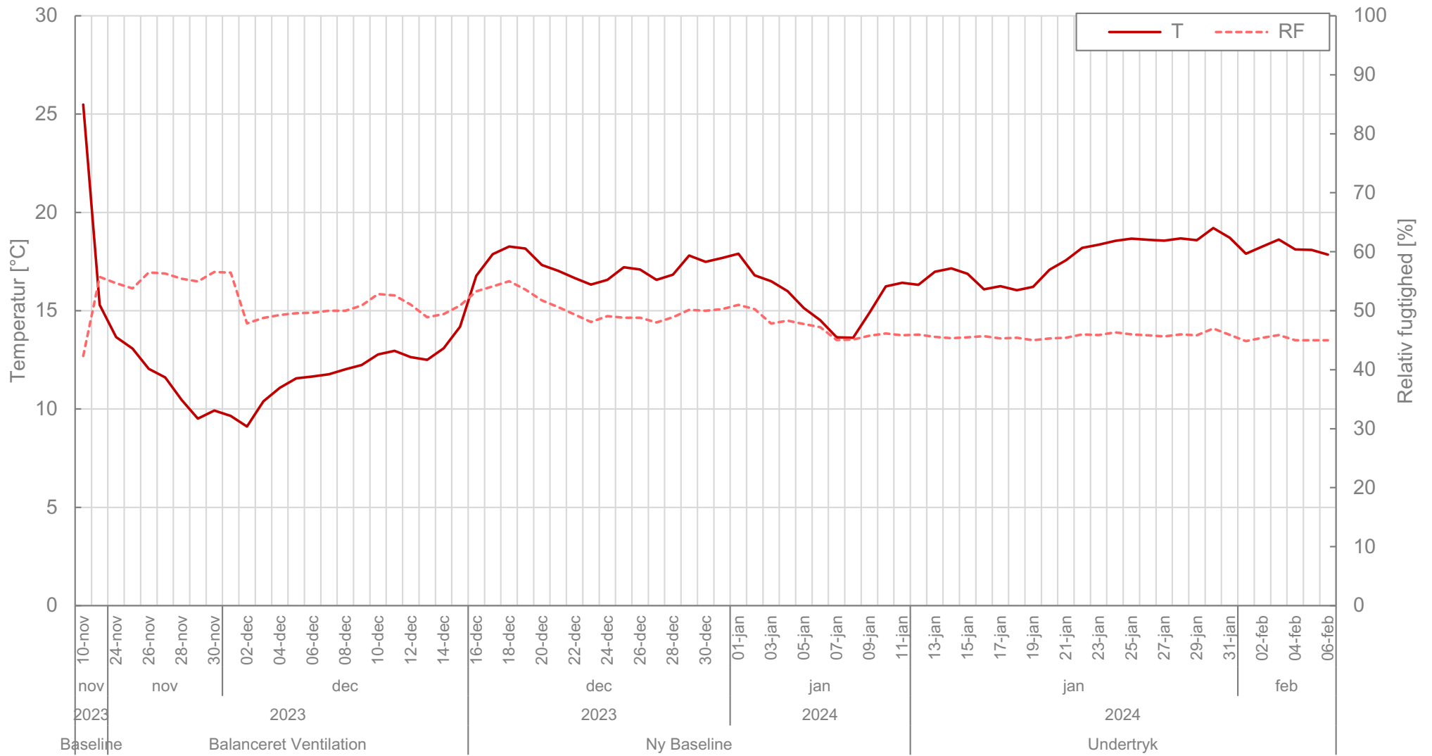
Bilag 16: Smartlogger (SL1) Træfugt på gulv ved T6 10/11 2023 til 5/2 2024
