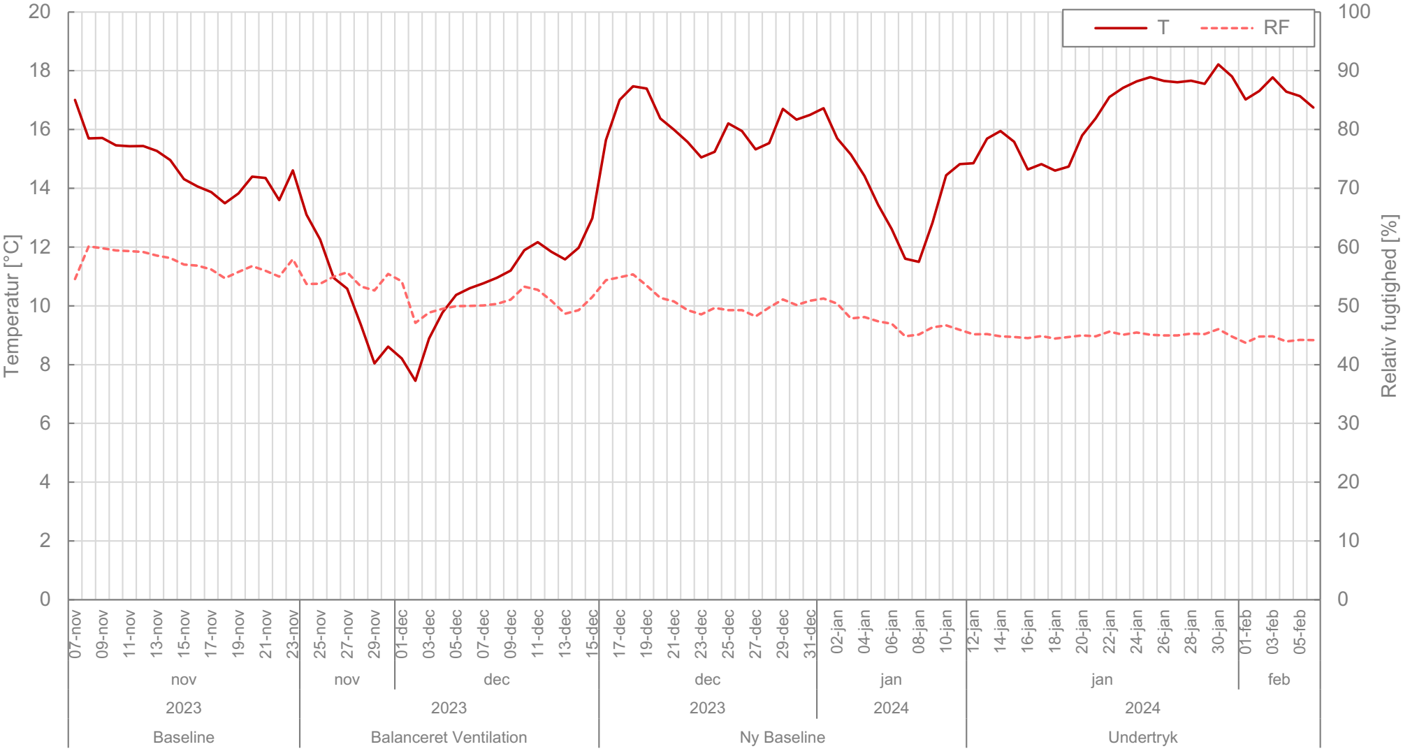
Bilag 11: T9 (ARH-1-23) - Temperatur og fugt på gulv 7/11 2023 til 5/2 2024
