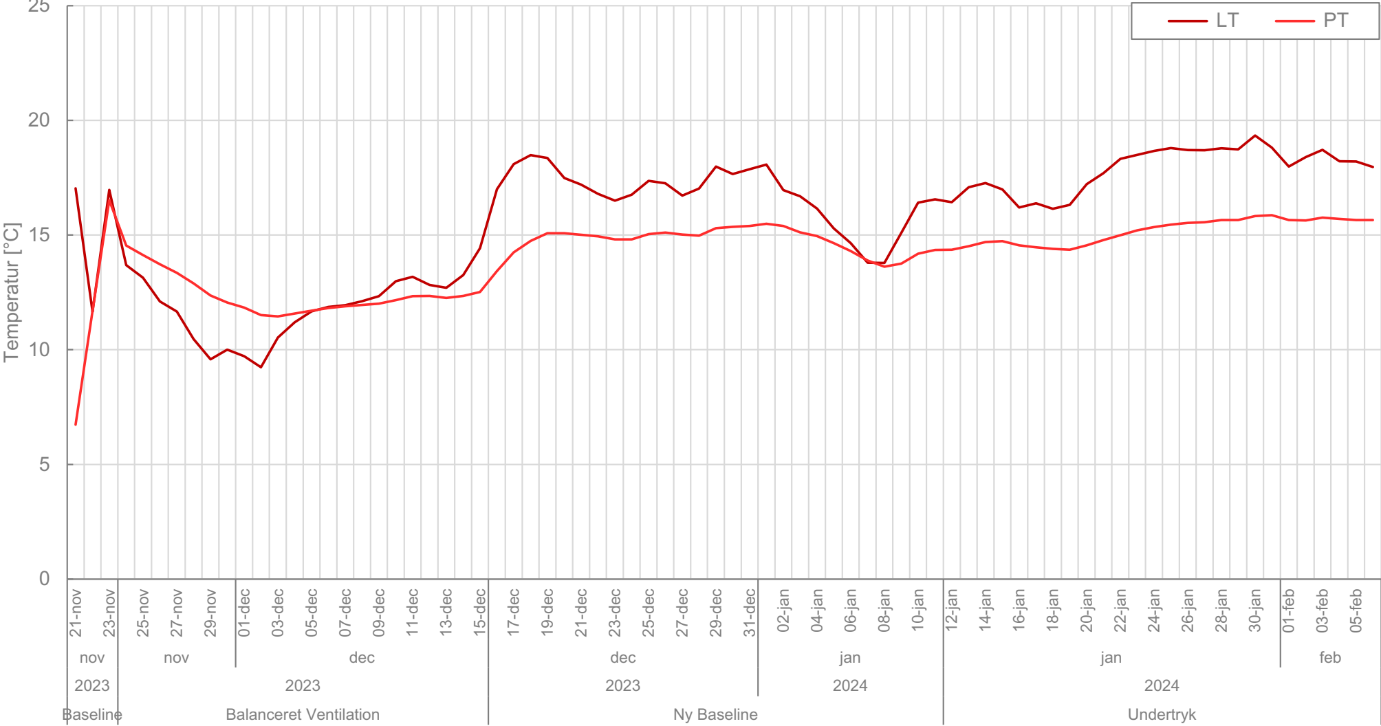
Bilag 8: T6 (V10-28) - Temperatur på og under gulv 23/11 2023 til 5/2 2024
