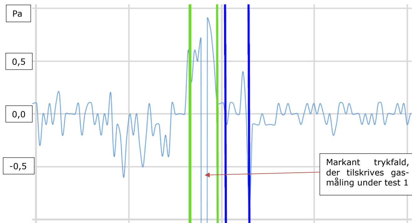
Figur 3: Differenstrykkurve for MP1004 i køkkenet. Test 1 ses mellem de to grønne, lodrette streger. Se bilag 3.
