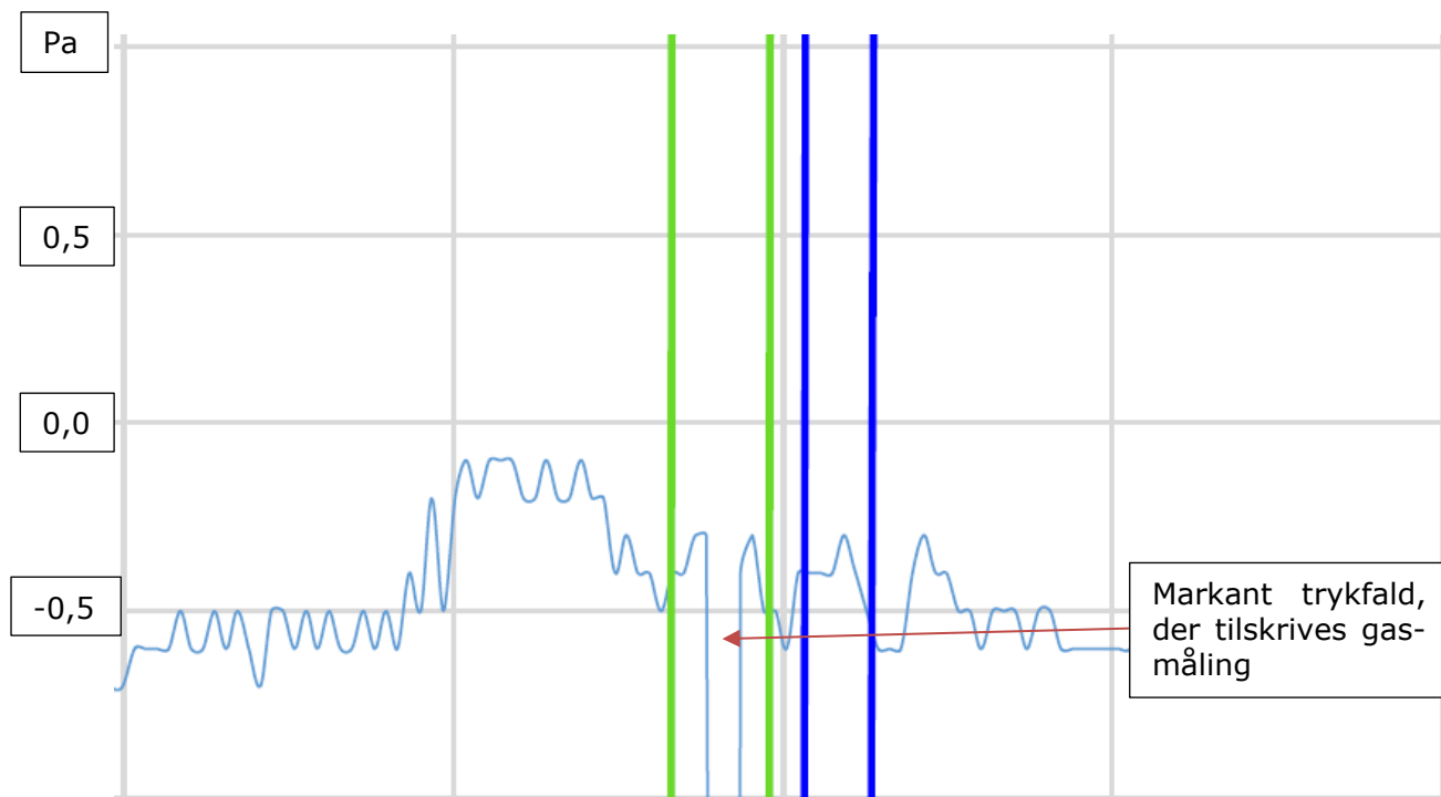
Figur 4: Differenstrykkkurve for MP1006 i gangen. Test 1 ses mellem de to grønne, lodrette streger. Se bilag 3.
