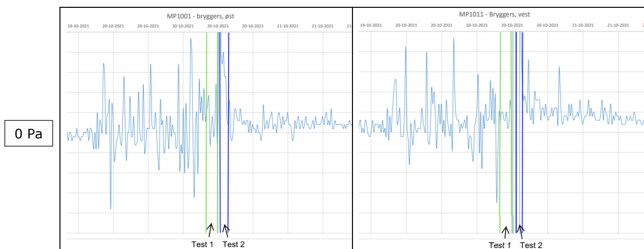
Figur 4: Differenstrykcurver for MP1001 og MP1011 i bryggers. Test 2 ses mellem de to mørkeblå, lodrette streger, bilag 3.
