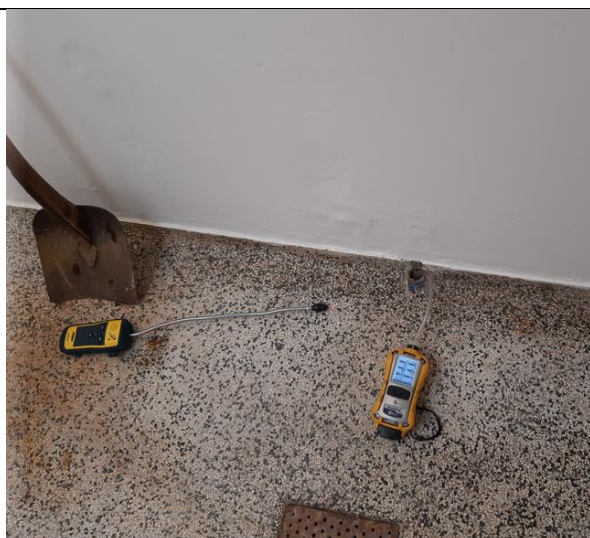
Foto 8: Markant indtrængningspunkt ved test 2 (P9), som er et metalrør.
