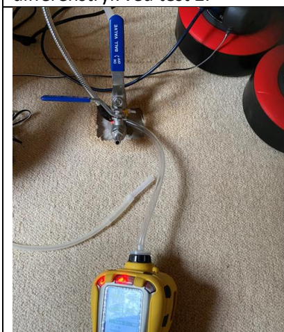
Foto 11: Nærbillede MP1003, ved måling ved gennemførelse ses påvirkning ved test 2.
